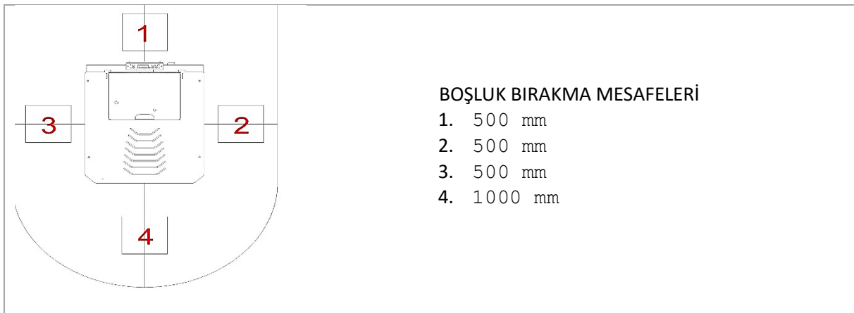
SOBA KURULUM ŞEMASI (ÜST GÖRÜNÜM) ŞEKİL
