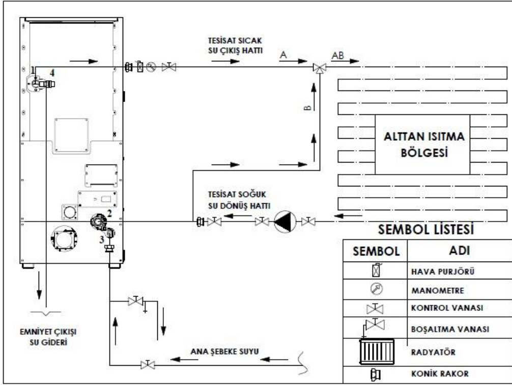
YERDEN ISITMA TESİSAT ŞEKİL (2)
