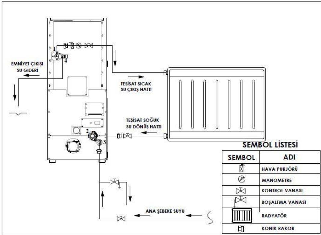
PANEL RADYATÖRLÜ TESİSAT ŞEKİL (1)
